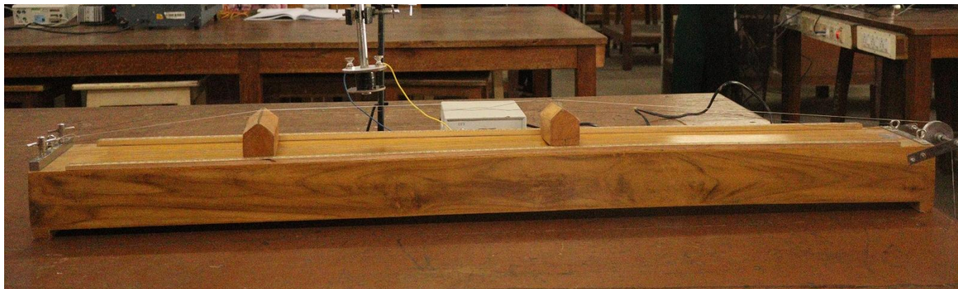
Sonometer
